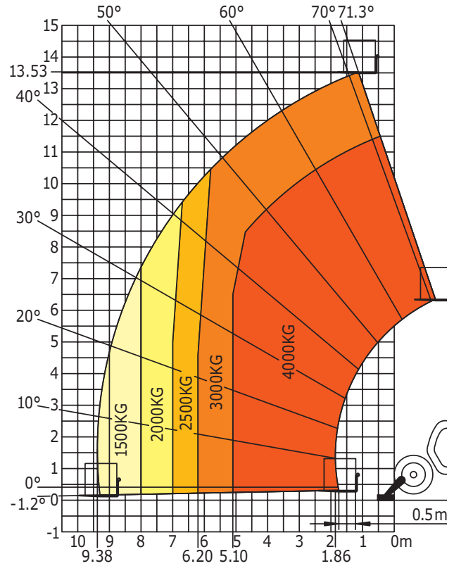
Machine sur stabilisateurs avec fourches CDG 500 mm
